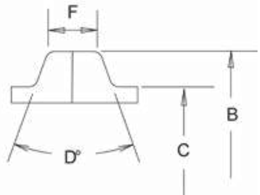
Ferrule
