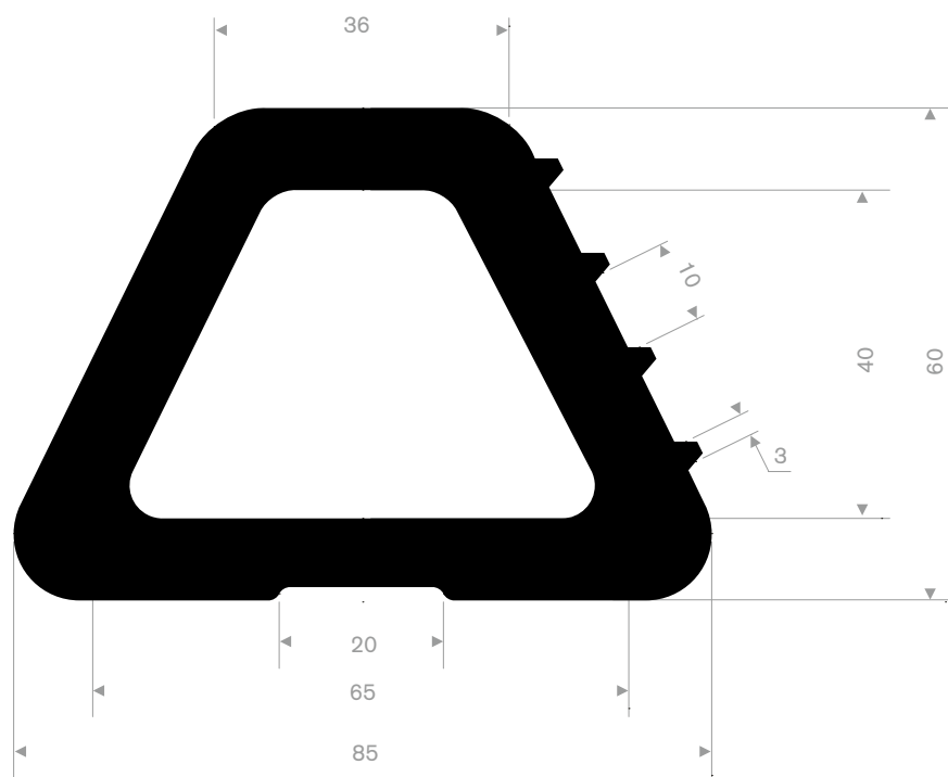
EPDM 70° Shore black roll length 12,5 meter
