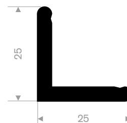
EPDM 60° Shore black roll length 50 meter
