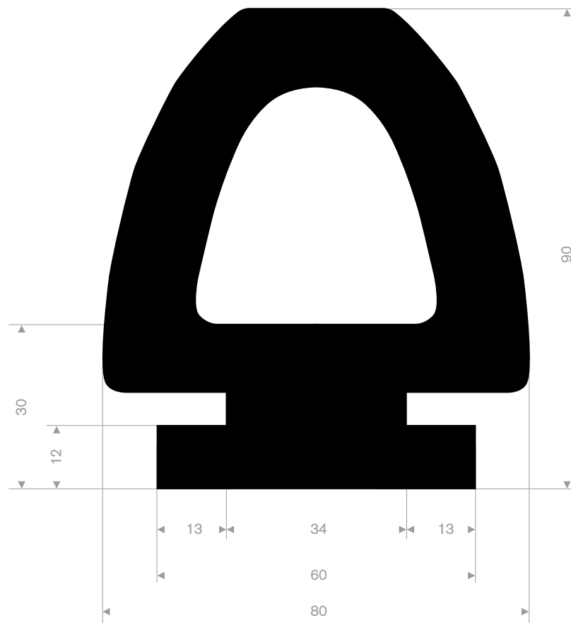
EPDM 70° Shore length 0,40 meter
